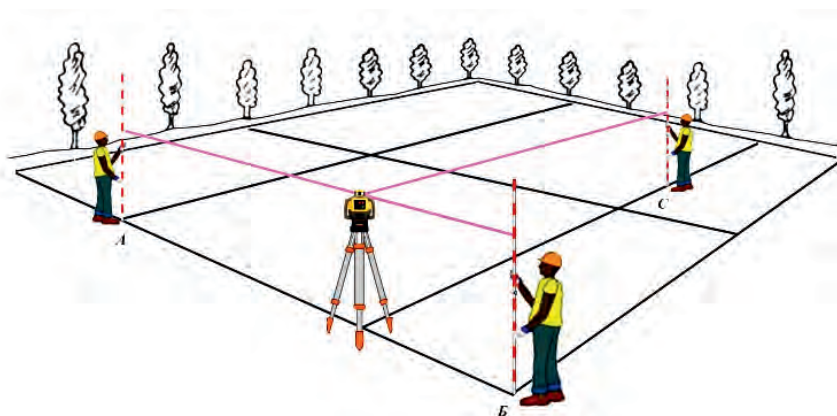
13-расм. Квадратлар ясашда тўғри бурчакни ҳосил қилиш
