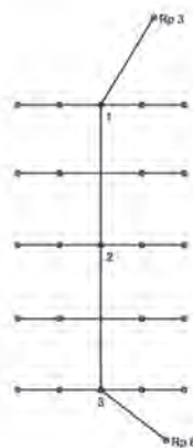
16-расм. Юзани магистраллар усулида нивелирлаш схемаси
