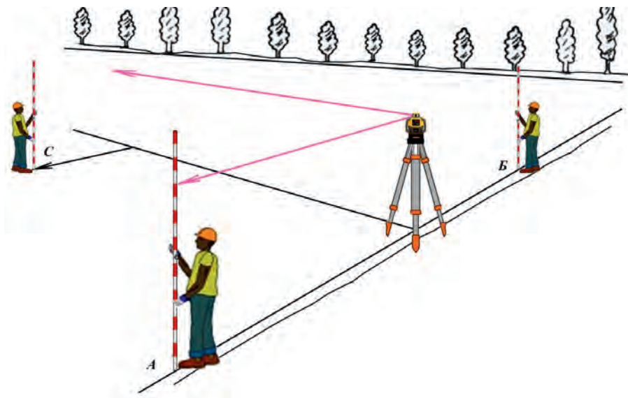
15-расм. 90^\circ бурчакни текшириш ишлари
